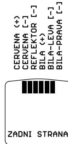
(b) Schéma zapojení
